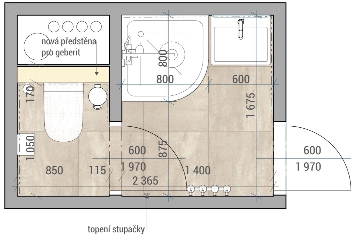
KOUPELNA VAR.1
