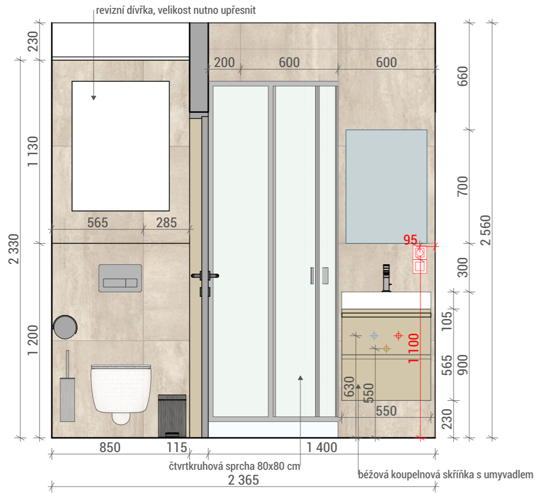
POHLED A
