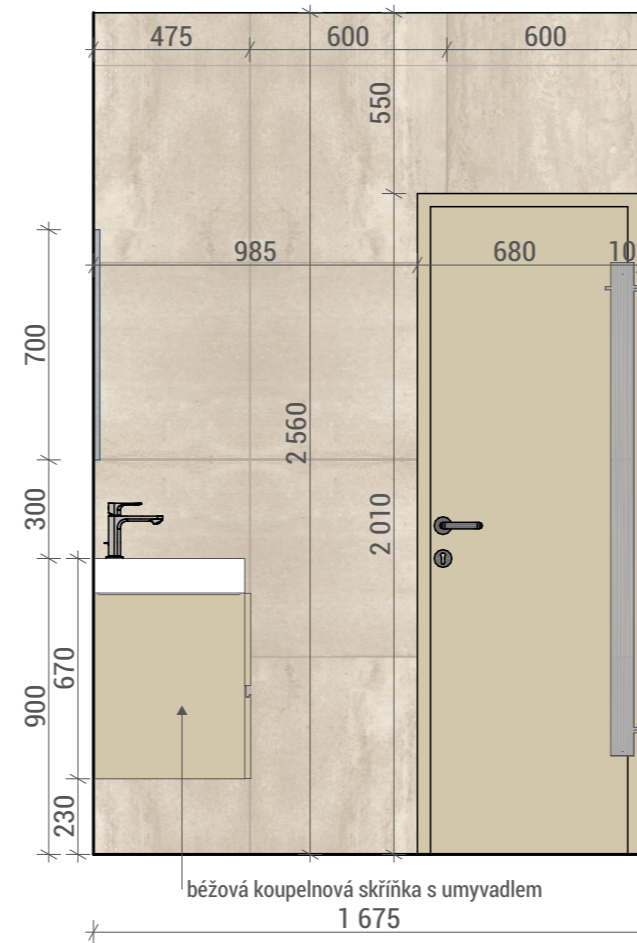
POHLED B1
