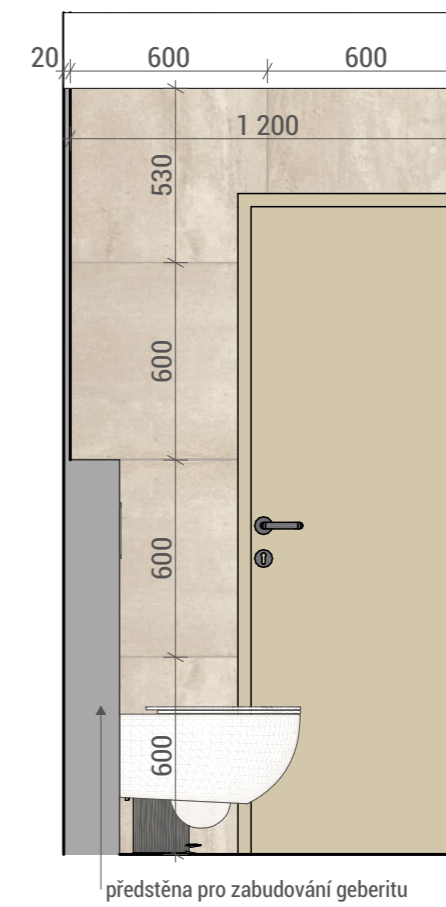
POHLED B2
