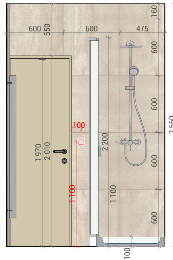
POHLED D1
