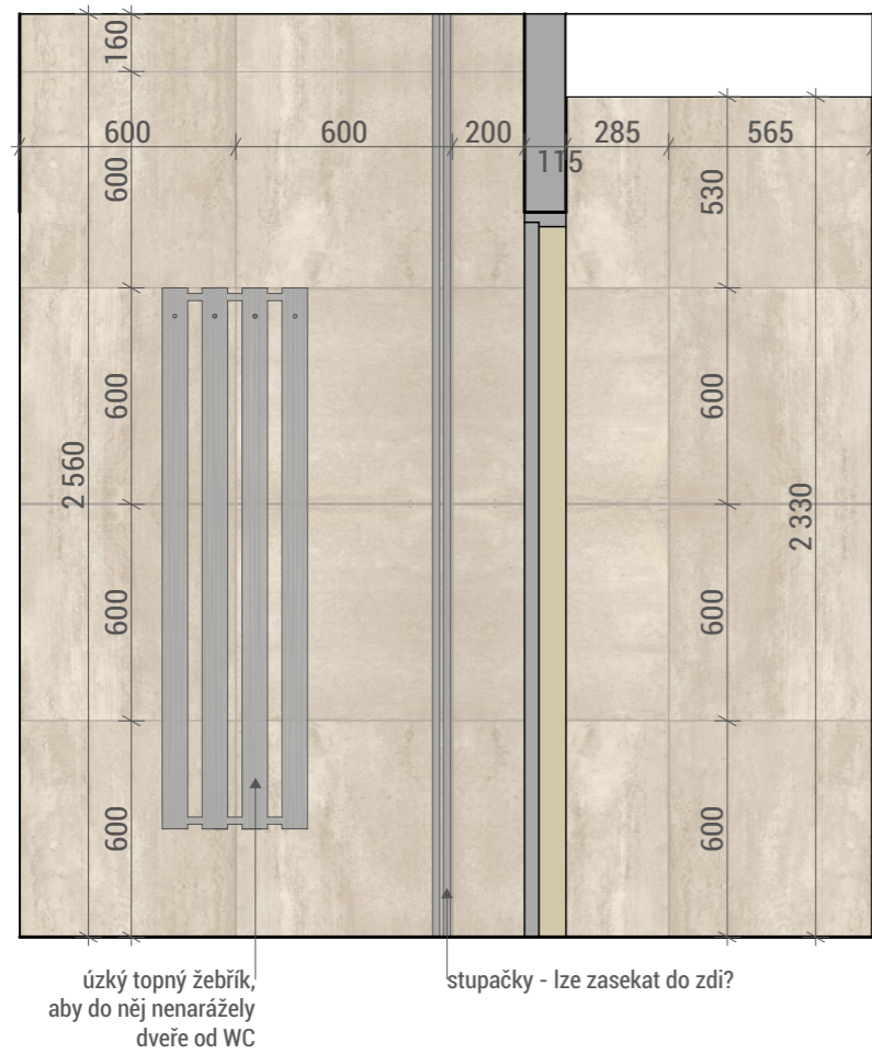
POHLED C
