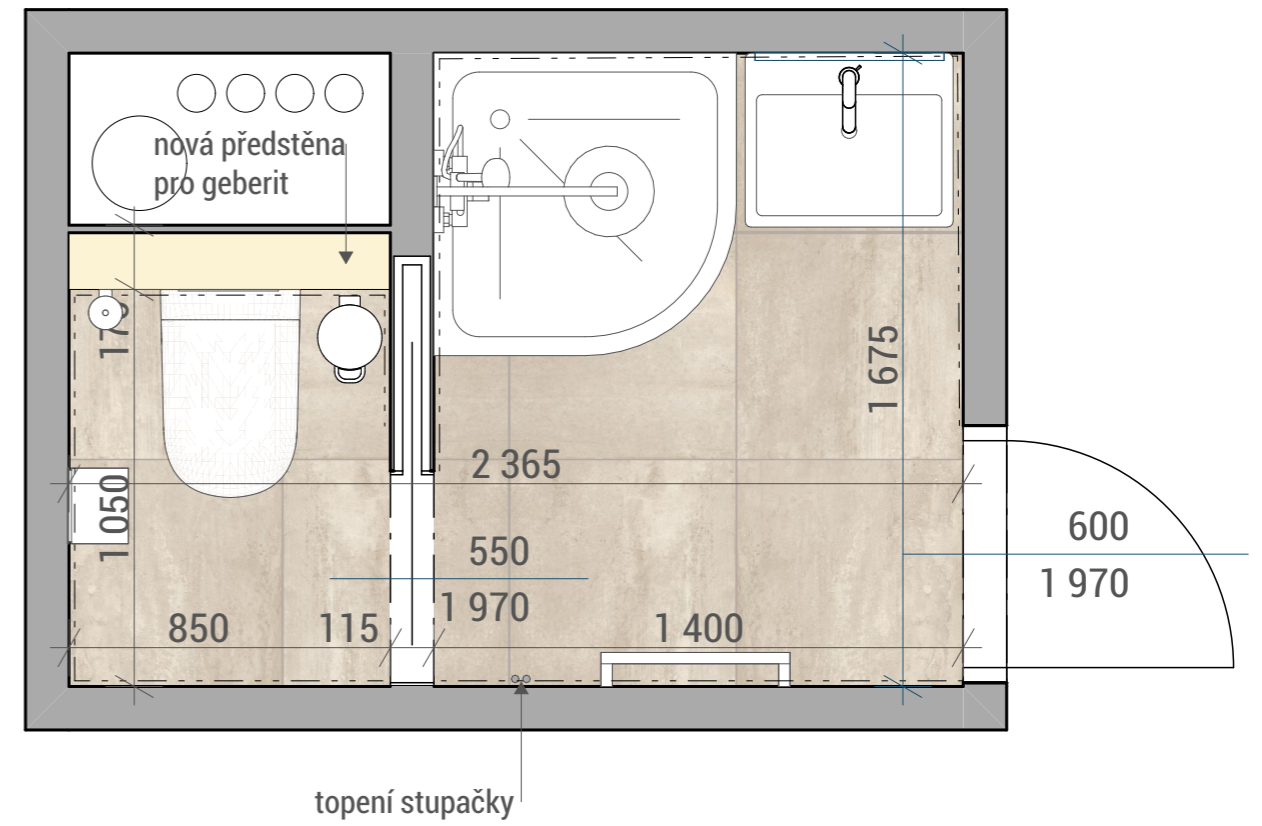
KOUPELNA VAR.2 (posuvné dveře v pouzdře)
